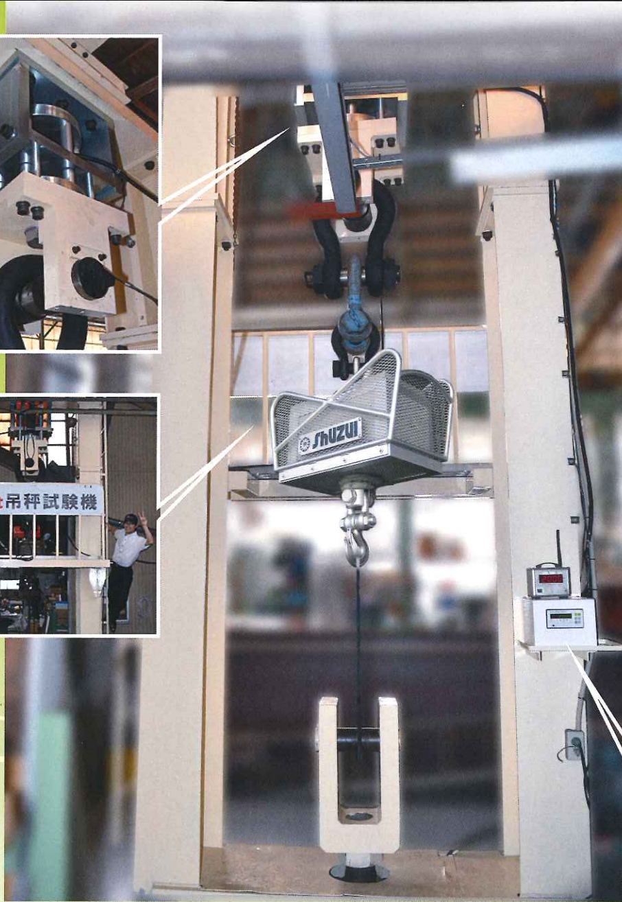
50t 吊秤試験機
